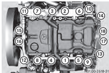
4R 1000 的紧固顺序
