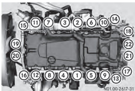
6R 1000 的紧固顺序
