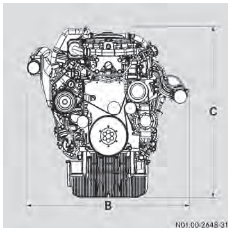
示例：发动机宽度和高度
