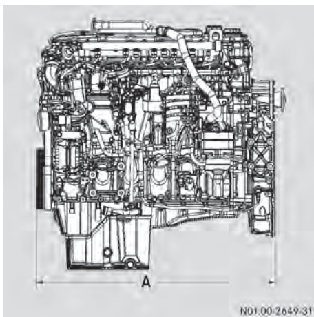
示例：发动机长度
