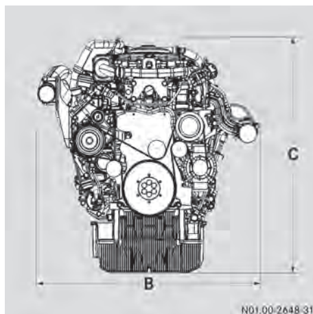
Larghezza e altezza del motore (esempio)
