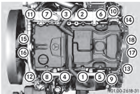
Schema di serraggio motore 4R 1000
