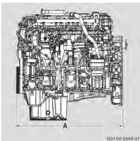
Lunghezza del motore (esempio)
