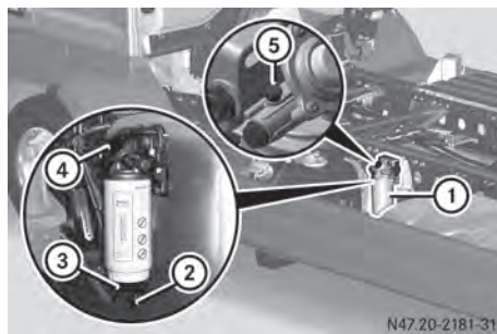
Prefiltro del carburante sull'autotelaio (esempio)
