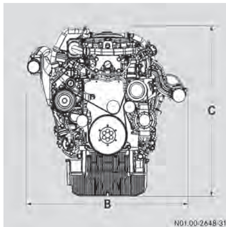
Anchura y altura del motor (ejemplo)
