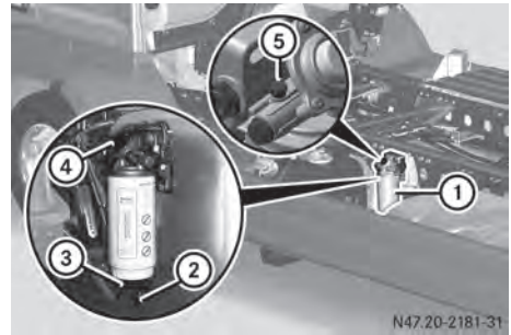
Prefiltro de combustible en el bastidor del chasis (ejemplo)
