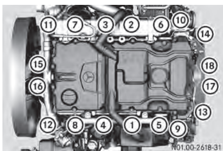
Esquema de apriete 4R 1000
