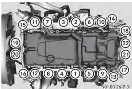
Esquema de apriete 6R 1000
